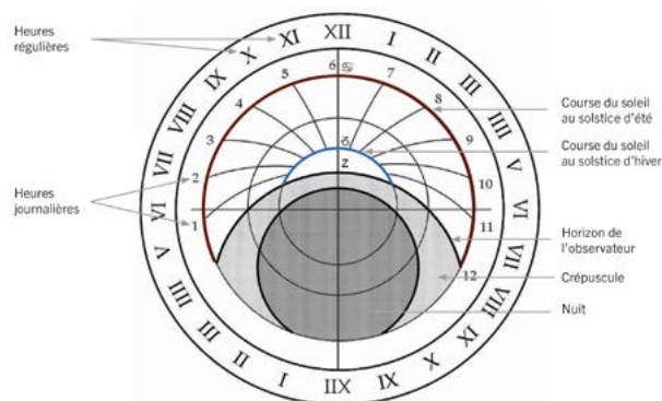
Figure 1 : le cadran de la Zytglogge
